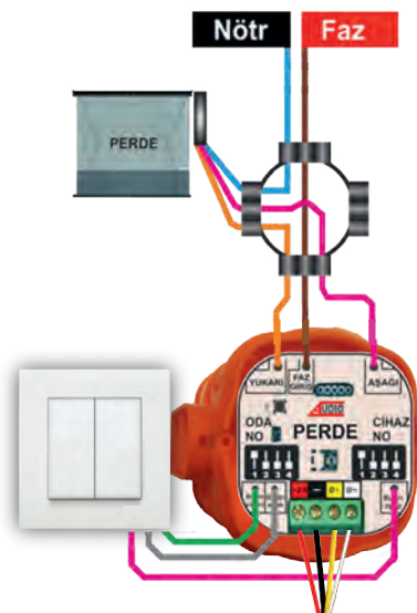
PERDE BAĞLANTISI
