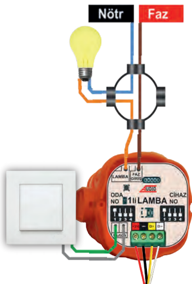
1'li LAMBA BAĞLANTISI
