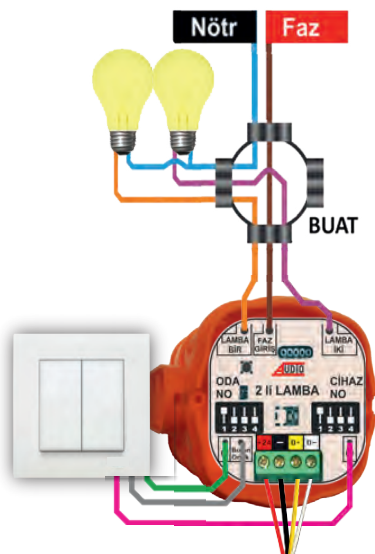
2'li LAMBA BAĞLANTISI
